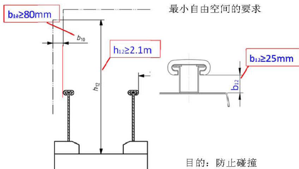
图 9、扶手带外缘距离尺寸示意图
